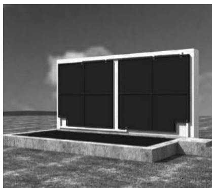
Bagvæggen i drivhuset består af varmeabsorberende, sortlakerede metalplader.
