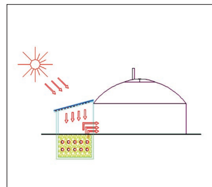
Den opsamlede varme gemmes i jorden til senere brug.
